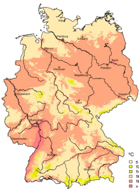
Lufttemperatur Sommer 2020 Temperature Summer 2020
