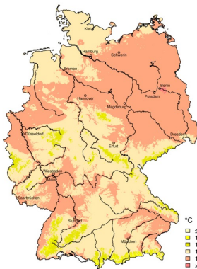
Lufttemperatur Sommer 2021 Temperature Summer 2021
